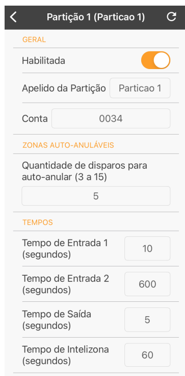
Figura 84: Parâmetros gerais, auto anulação e temporização
