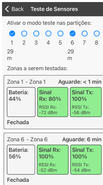
Figura 101: Aba do modo de teste de sensores
