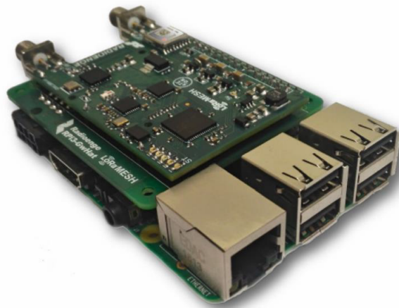
Figura 7: Gateway LoRa acoplado ao Raspberry Pi 3
