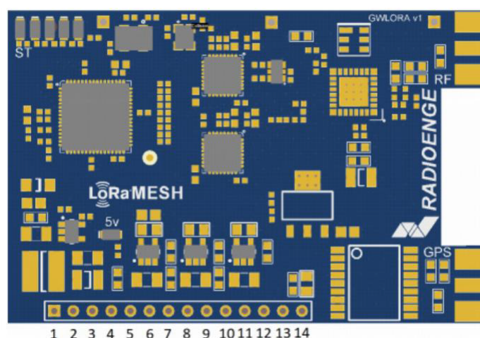
Figura 3: Pinout
